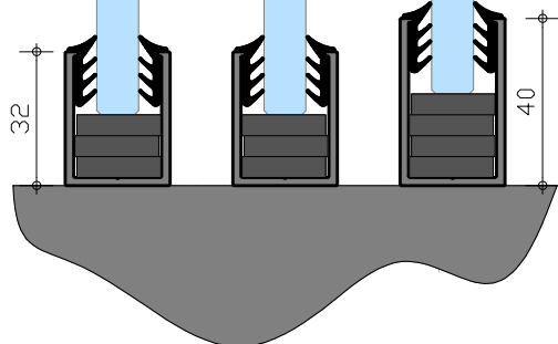
Detail B vloer aansluiting
